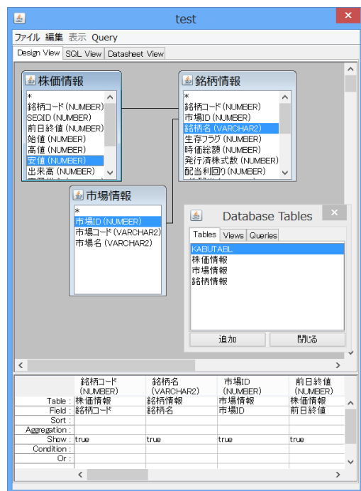
クエリビルダ
